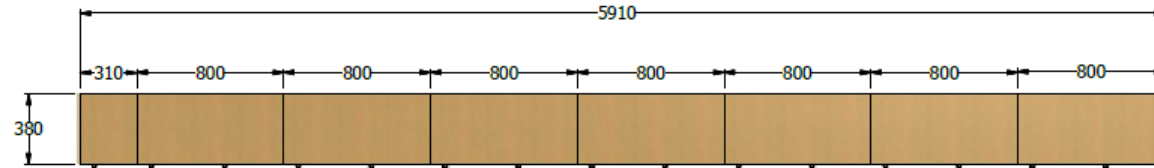
vista superior
